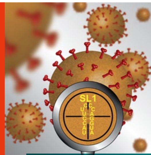
La structure SL1 du -CoV-2, une cible thérapeutique pour bloquer le virus © F. Martin
