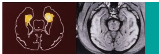
Tomographie du cerveau par émission de positrons (TEP) et résonance magnétique (RMN).
