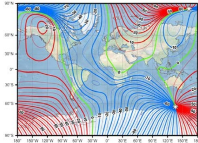
L'association internationale de géomagnétisme et de géophysique, à laquelle contribuent les géophysiciens alsaciens, a mis à jour le modèle du champ de référence géomagnétique international (IGRF). © Earth Planets Space
