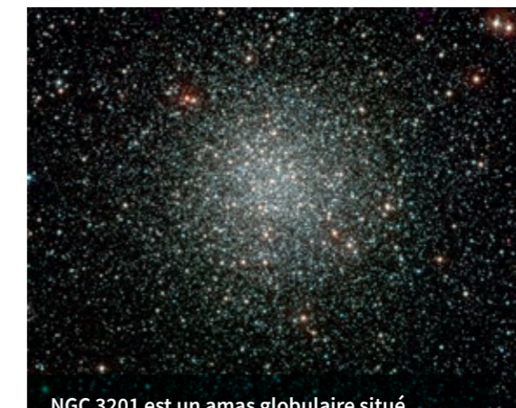
NGC 3201 est un amas globulaire situé à 16 000 années-lumière du Soleil.
